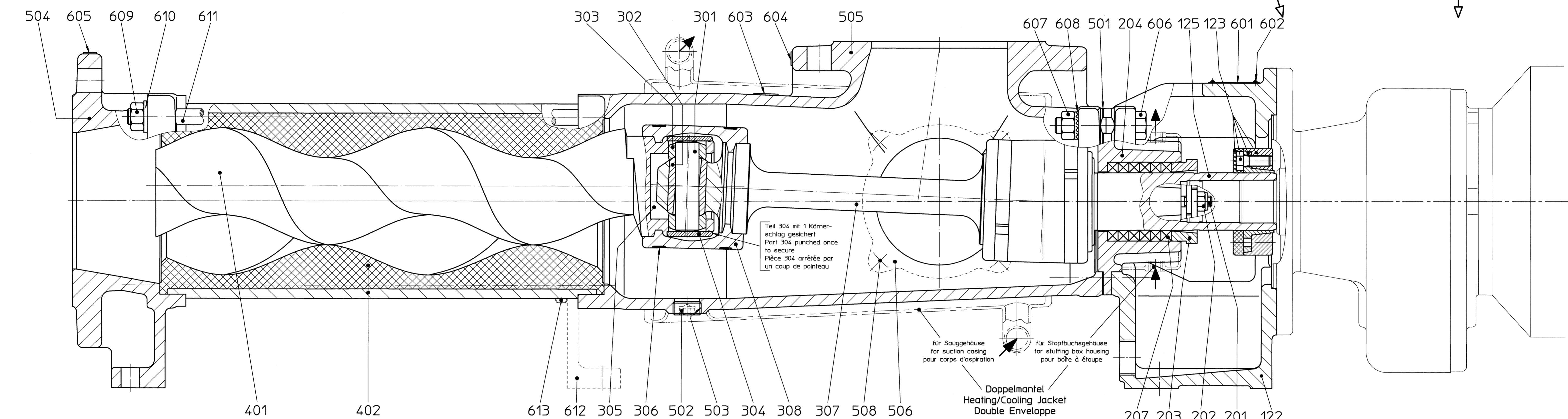
Pumpe in Grundausführung Standard Type Pump Pompe Type Standard
